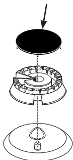
Tapa del Quemador Redondo (Extraíble)
